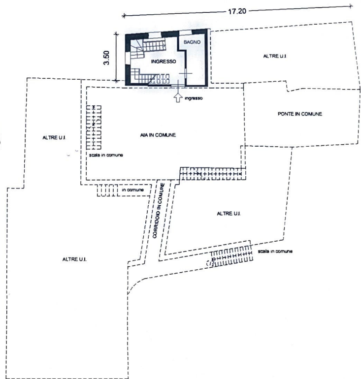
PIANO PRIMO (P1) H max = 2.45 m
