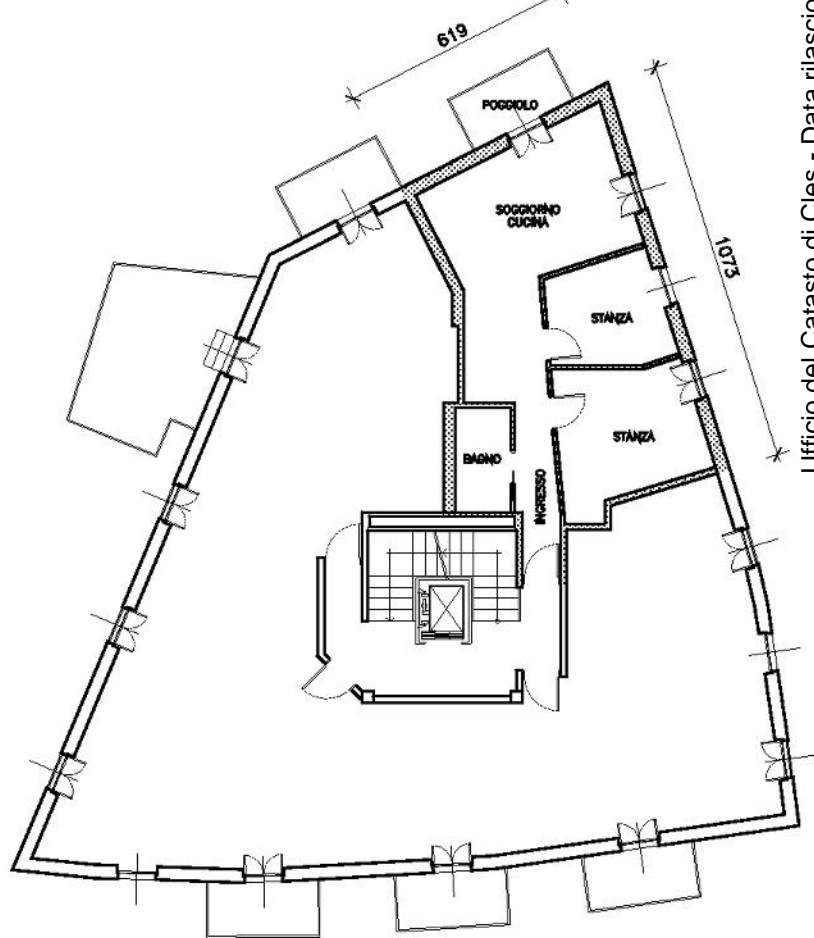
PIANTA PIANO PRIMO H = 2.45 m.
